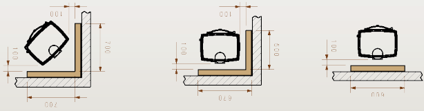
Utenpåliggende brannmur
